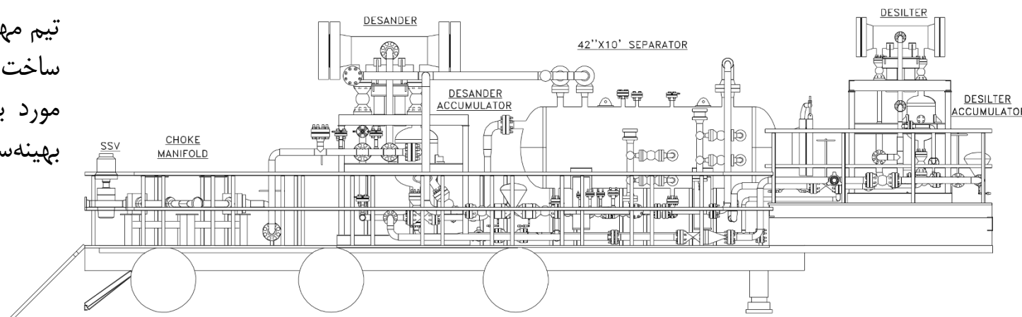
SEPARATOR & DESANDER
