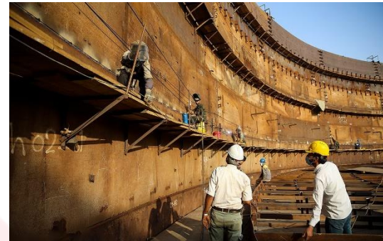
تأمین و همکاری در تولید ۱۲,۰۰۰ تن ورق A516Gr.70 +N عسلویه پروژه مخازن سبز
